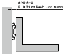
■ 安装间隙
