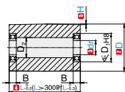
圆弧形 BFSDC
