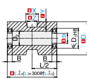
肋槽型 BFSDR
