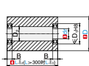
直柱型 BFSDD
