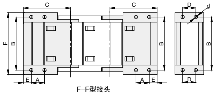
F-F型接头
