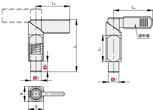
PKHWA 焊接型 ( A )
