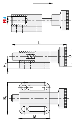
PKPHN 有头无卡锁
