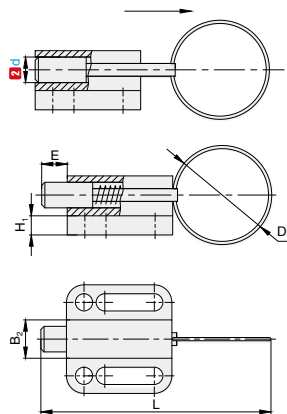
PKPCN 有环无卡锁
