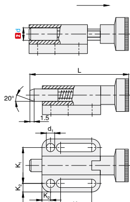
PKPHL 有头有卡锁
