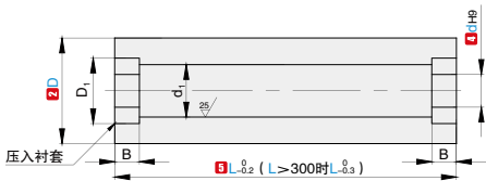
RTMRC 芯材
