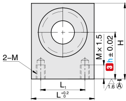
BBM 底座安装型
