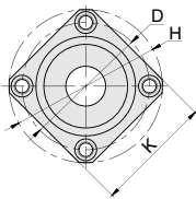
BDELD K 方型
