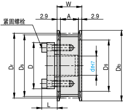
SEHF 标准型
